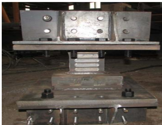
Figura 1. Fotografía de un disipador SLB ( Shear Link Bozzo ).
