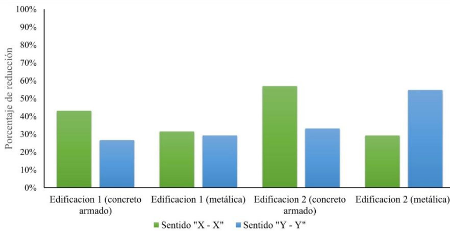
Figura 13. Análisis comparativo de desplazamientos máximos de piso de los edificios 1 y 2.
