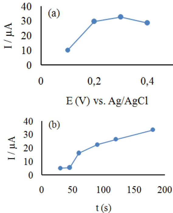
Figura 2. a) Corriente de pico vs. Potencial (V) de preconcentración. b) Corriente de pico vs Tiempo de preconcentración (s). Potencial de preconcentración -0,30 V. Concentración de As(III) 10 \mu\text{g L}^{-1} . Redisolución por SWV: E_i = -0,40 V; E_f = 0,40 V; Amplitud = 75 mV, Ancho = 50 ms; Frecuencia = 600 Hz.
