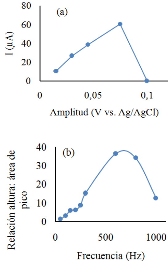
Figura 3. a) Corriente de pico vs. Amplitud del pulso. b) Relación entre la altura: área de pico vs. Frecuencia de imposición de potencial de onda cuadrada. Concentración de As(III) 10 \mu\text{g L}^{-1} . Potencial de preconcentración -0,30 V, Tiempo de preconcentración 180 s. Redisolución por SWV: E_i = -0,40 V; E_f = +0,40 V; Ancho = 50 ms.
