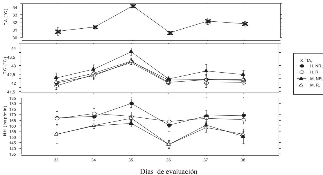
FIGURA 1. VARIACIONES PROMEDIO DE LA TEMPERATURA CORPORAL (TC) Y DEL NIVEL DE HIPERVENTILACIÓN, SEGÚN CAMBIOS DE LA TEMPERATURA AMBIENTE (TA) A LO LARGO DE EXPERIENCIA 1 (EXP. 1) Y DURANTE LA ÚLTIMA SEMANA DE LA EXPERIENCIA 2 (EXP. 2) DURANTE LOS DIFERENTES DÍAS DE EVALUACIÓN, SEGÚN TRATAMIENTO DE RESTRICCIÓN DE ALIMENTO (NR = NO RESTRINGIDO Y R = RESTRINGIDO) Y SEXO DE LOS POLLOS (H= HEMBRA Y M = MACHO)/ VARIATIONS MEDIATE OF THE CORPORAL TEMPERATURE (TC) AND OF THE LEVEL OF HIPERVENTILATION, ACCORDING TO CHANGES OF THE TEMPERATURE ENVIRONMENT (TA) ALONG EXPERIENCE 1 (EXP. 1) AND DURING THE LAST WEEK OF THE EXPERIENCE 2 (EXP. 2) DURING THE DIFFERENT DAYS OF EVALUATION, ACCORDING TO TREATMENT OF FOOD RESTRICTION (NR = NOT RESTRICTED AND R = RESTRICTED) AND SEX OF THE CHICKENS (H = FEMALE AND M = MALE).
