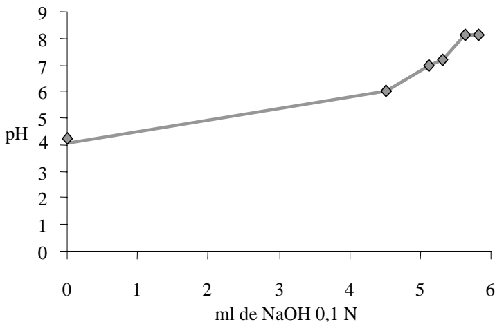
Figura. 1. Curva de neutralización de los ácidos orgánicos de la pulpa de guayaba ( Psidium guajava L) del tipo “Criolla Roja”.
